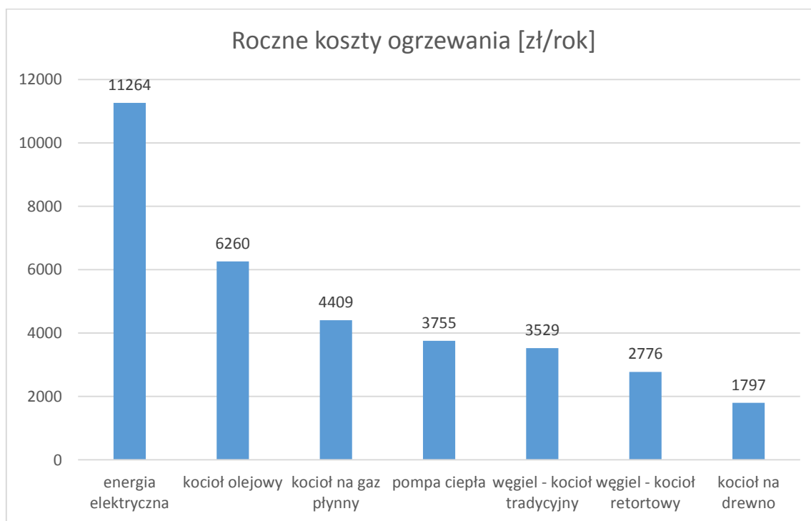
Rysunek 19 Porównanie rocznych kosztów wytworzenia energii w odniesieniu do jednostkowych wskaźników kosztów energii dla różnych nośników energii
