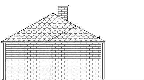
ELEWACJA ZACHODNIA 1:100
