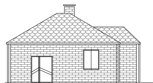
ELEWACJA POŁNOCNA 1:100
