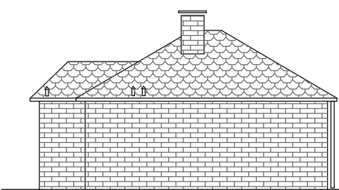
ELEWACJA POŁUDNIOWA 1:100
